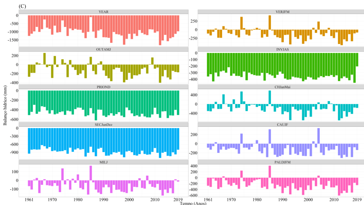
Figura 3. Comportamento da precipitação l (A), da evapotranspiração de referência (B) e do balanço hídrico climático (C) para os subperíodos: anual, verão, outono, inverno, primavera, período chuvoso, período seco, plantio caupi, plantio milho e plantio palma, de 1912 a 2019 (A) e de 1961 a 2019 (B e C).
